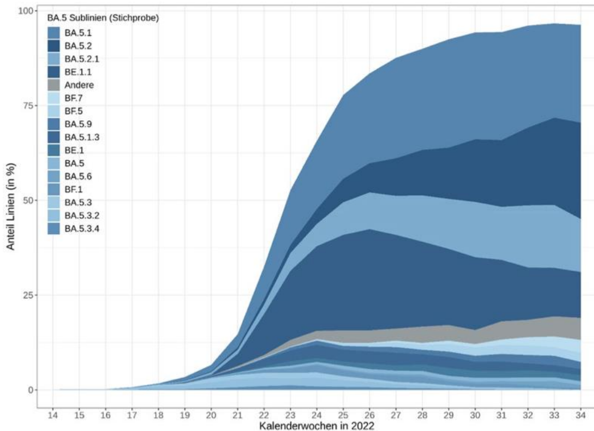
Abbildung 2–5 Prozentuale Anteile der Omikron-BA.5 Sublinien mit einem Anteil von jemals >1 %, bezogen auf die Genomsequenzen aus der Stichprobe, absteigend sortiert nach ihrem Anteil in KW 34/2022. Unter „Andere“ werden alle weiteren BA.5 Sublinien subsumiert, deren Anteil in der Stichprobe durchgehend \leq 1 % lag. Quelle: Wöchentlicher COVID-19-Lagebericht des RKI vom 8.9.2022, S. 28
