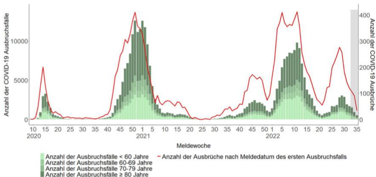
Abbildung 6–12: Gemeldete COVID-19-Ausbrüche in Alten- und Pflegeheimen mit mindestens 2 Fällen nach Meldedatum des ersten Ausbruchsfalls seit MW 10/2020. Die Ausbruchsfälle mit der Angabe <60 Jahre umfassen auch Besucherinnen und Besucher sowie Mitarbeitende der Einrichtungen. Datenstand 6.9.2022. Quelle: RKI. Wöchentlicher COVID-19-Bericht des RKI vom 8.9.2022, S. 8
