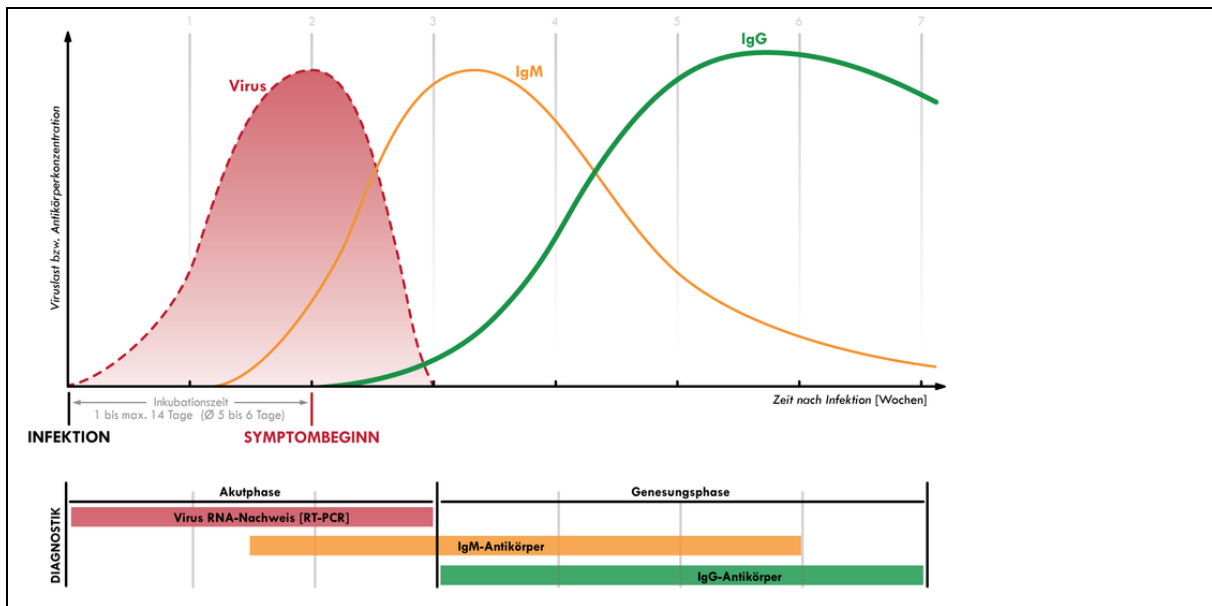
Abbildung 2–11: Viruslast, Diagnostik, Antikörper im Verlauf der Infektion.
