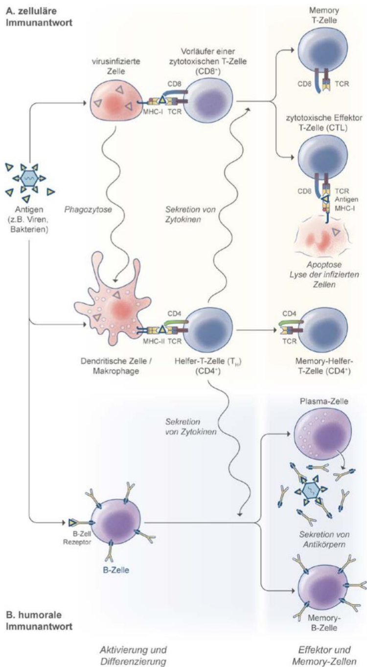
Abbildung 2-7: Zelluläre und humorale Komponenten des erworbenen Immunsystems.
