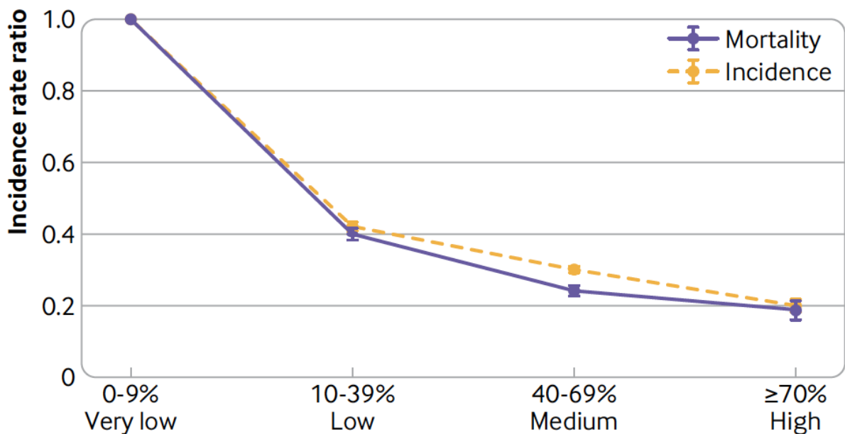
Abbildung 4–7: COVID-19-Mortalität und -Inzidenz (y-Achse) und Durchimpfungsrate (x-Achse). Quelle: Suthar et al. 27.4.2022
