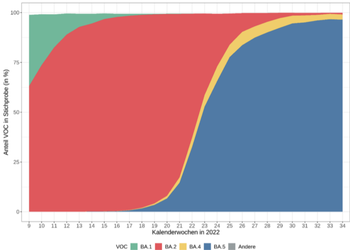
Abbildung 2–4: Prozentuale Anteile der VOC (einschließlich der jeweiligen Sublinien) mit einem Anteil von jemals >1% bis KW 34/2022. Quelle: Wöchentlicher COVID-19-Lagebericht des RKI vom 8.9.2022, S. 26
