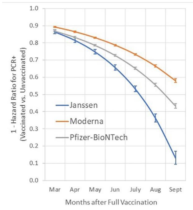
Abbildung 4–15: Impfeffektivität für SARS-CoV-2-Infektion für 3 Impfstoffe.
