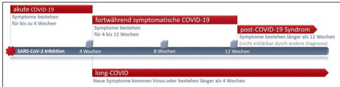
Abbildung 2–22: Überblick über COVID-19 Nomenklatur. Quelle: DGP 12.7.2021, S. 59, angelehnt an NICE
